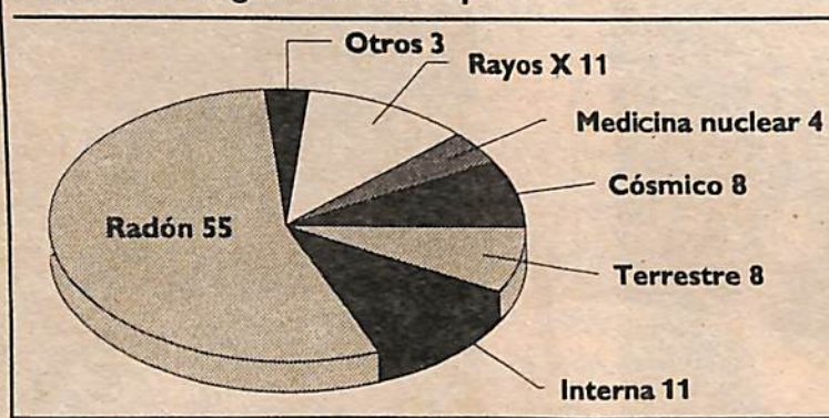
Porcentajes de radón y otras fuentes contaminantes naturales y artificiales, a las que están expuestas los habitantes de grandes metrópolis
