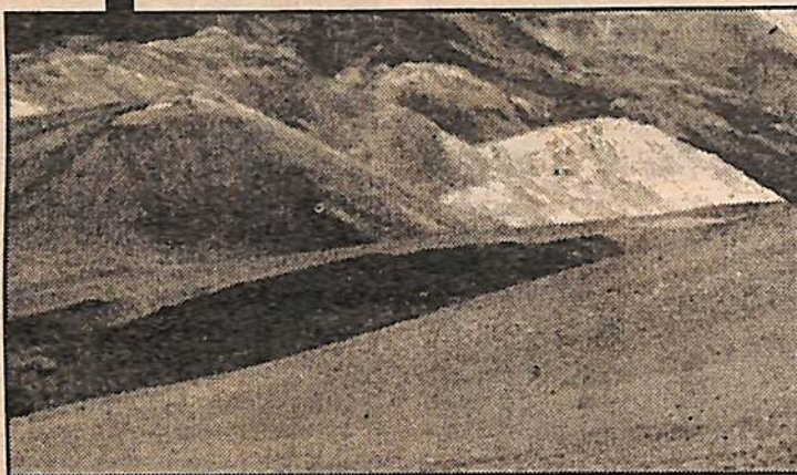
En terrenos graníticos, se presenta la mayor concentración de radón en estado natural
