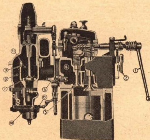
Corte trasversal donde se muestran los dientes elementos de nuevo organismo cambio de combustibles en el arranque.-
